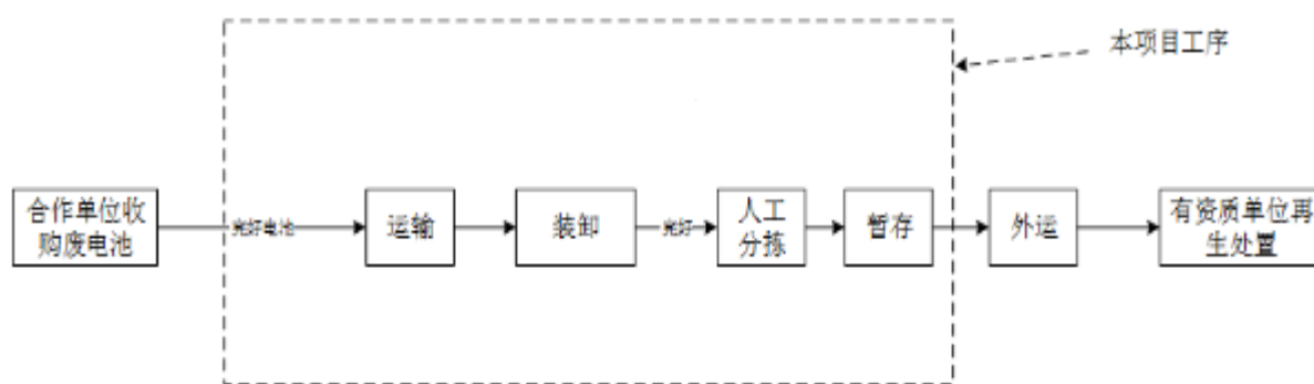
图5-1 项目工艺流程图
