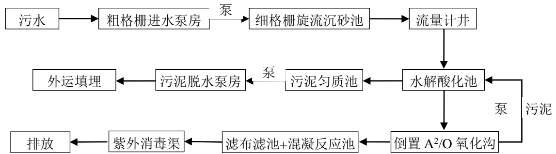
图 7-1 金风环保（沭阳）有限公司（原沭阳凌志水务有限公司）工艺流程图
